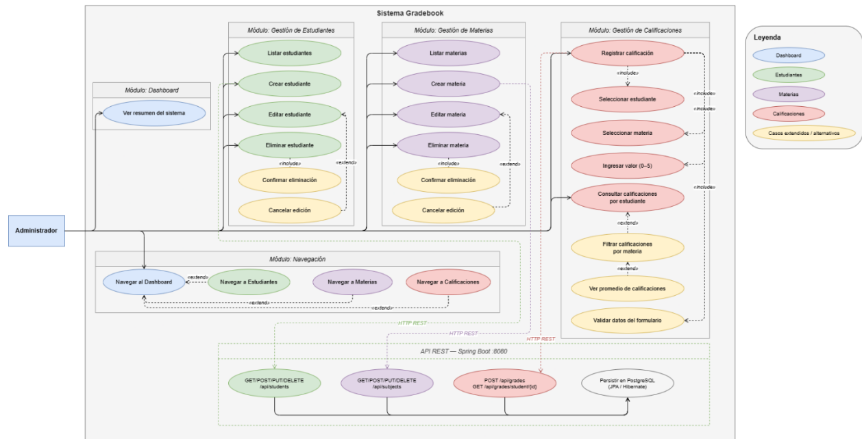
Diagrama de Casos de Uso — Gradebook
