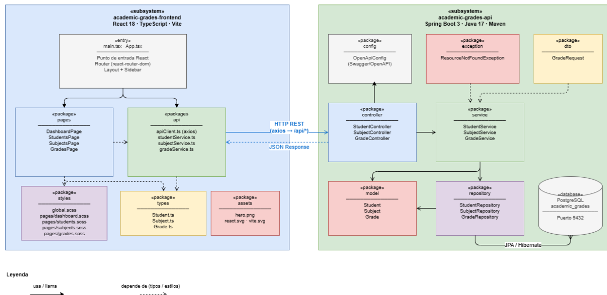
Diagrama de Paquetes — Gradebook
